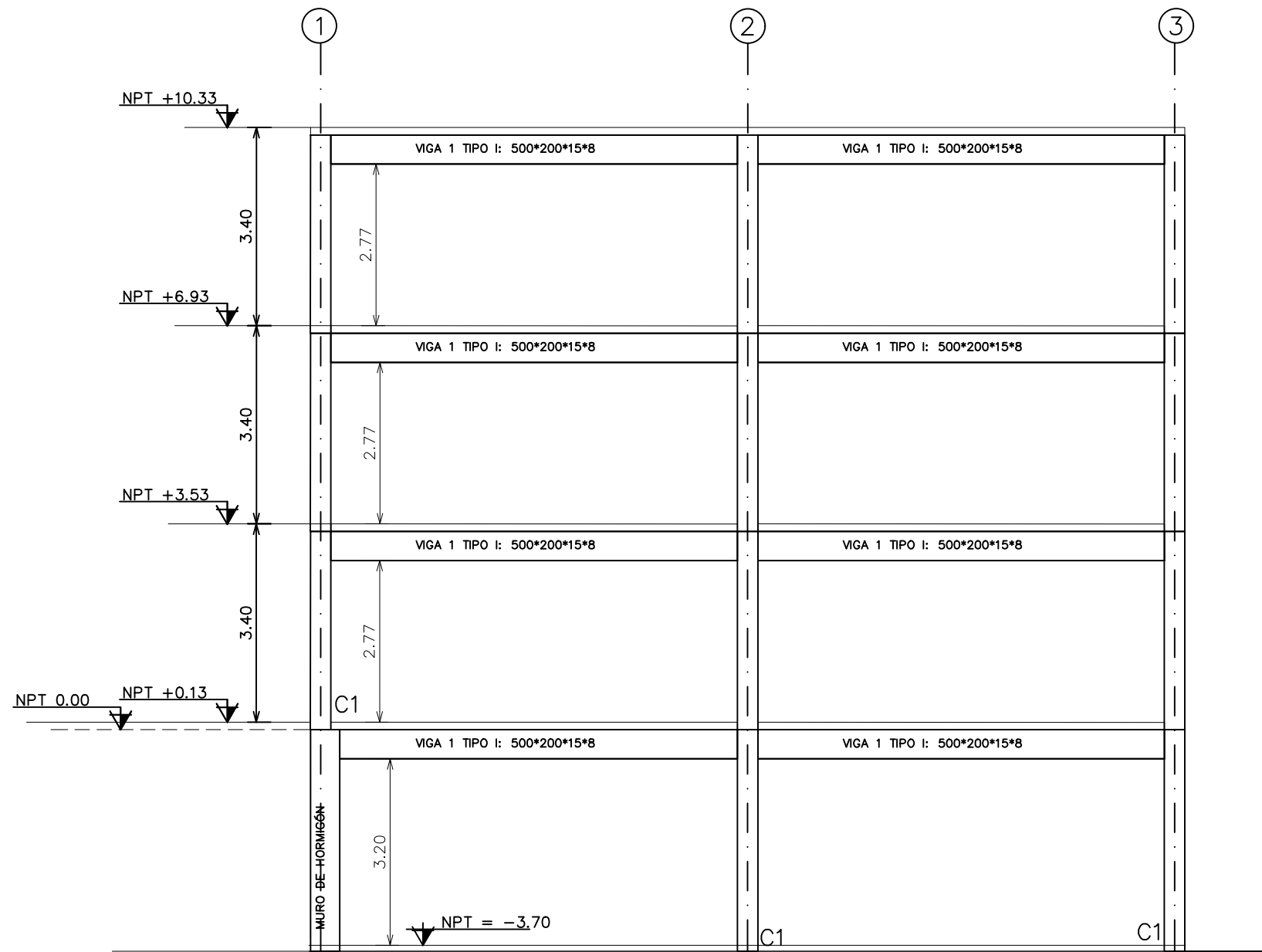
ELEVACIÓN EDIFICIO - EJE B Escala 1:100
