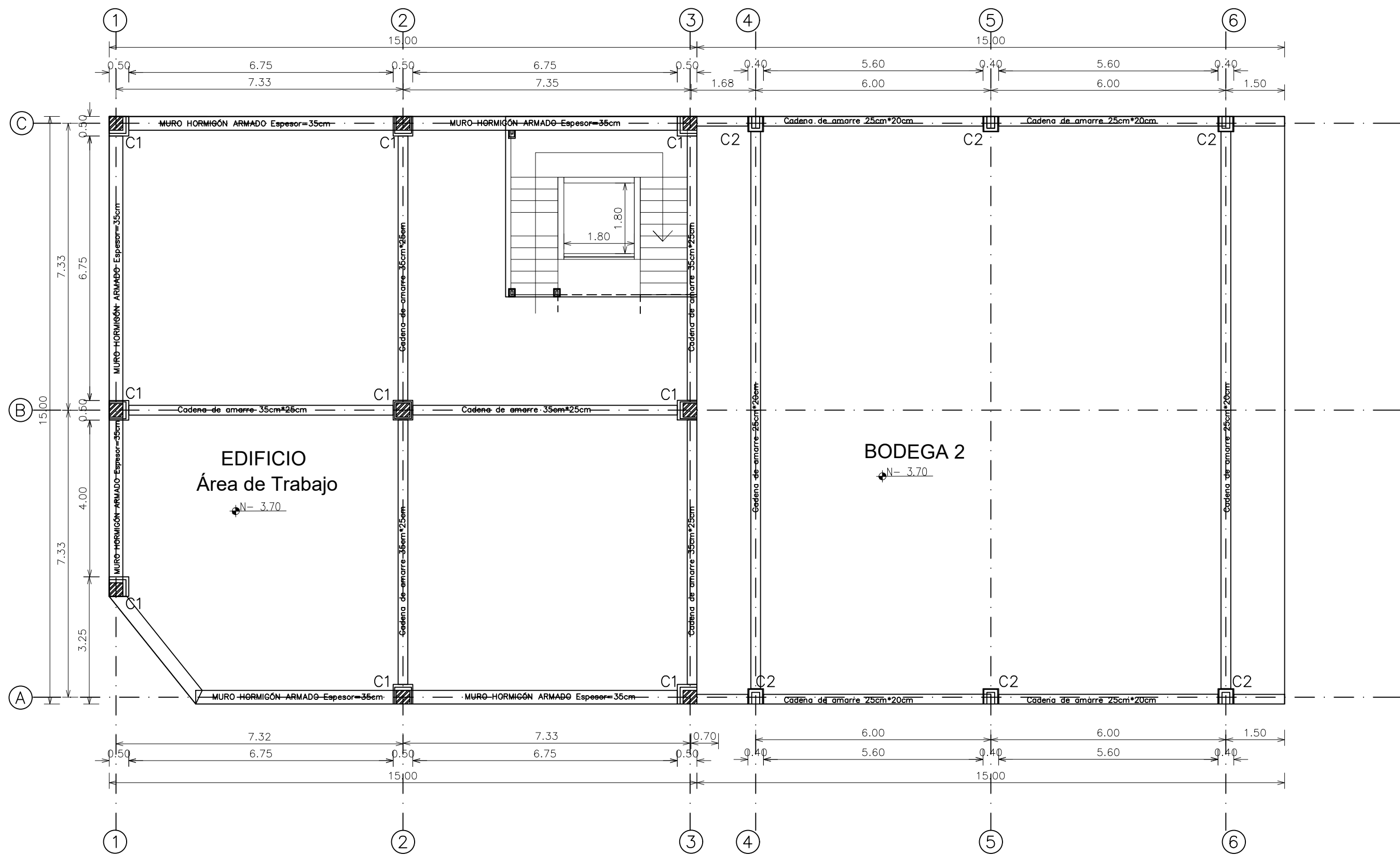
PLANTA COLUMNAS Escala 1:100
