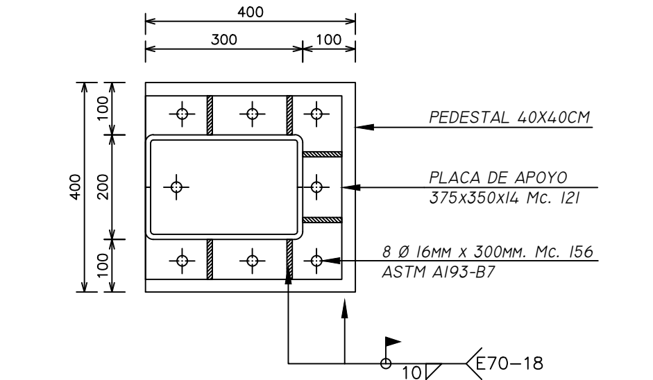
PLACA DE APOYO C2-( 6u ) Escala 1:10
