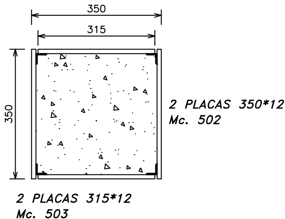
DETALLE COLUMNA C1 Escala 1:10
