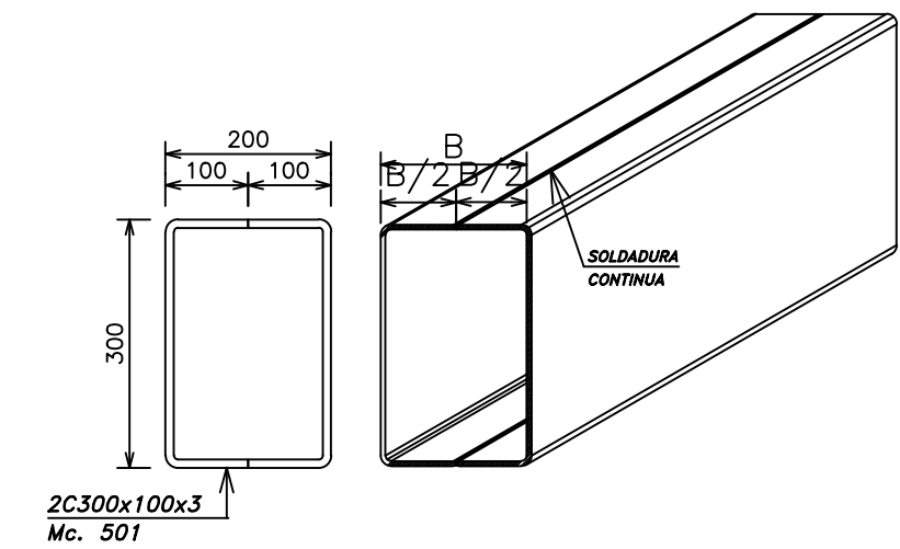
DETALLE COLUMNA C2 Escala 1:10
