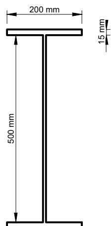
VIGA PRINCIPAL V1 Escala 1:10
