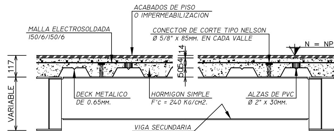
DETALLE SECCION TIPICA DE LOSETA Escala S:N
