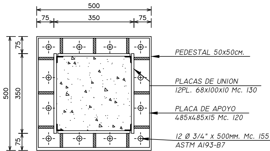
PLACA DE APOYO C1-CENTRAL Escala 1:10
